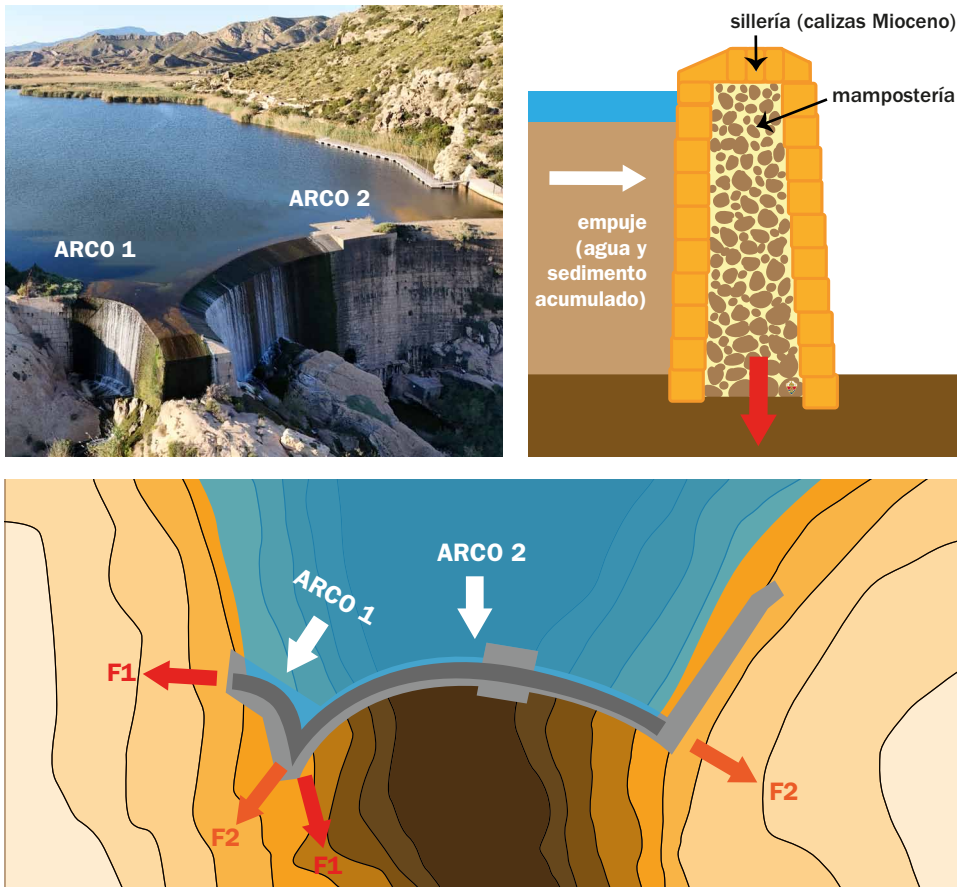
Figura 36. Planta y sección de la presa de Elche (modificado de Irles Más, R., Jaén i Urban, G. e Irles Más, F., 2000; La presa de Elche sobre el río Vinalopó. I Congreso Nacional de Historia de las Presas).
